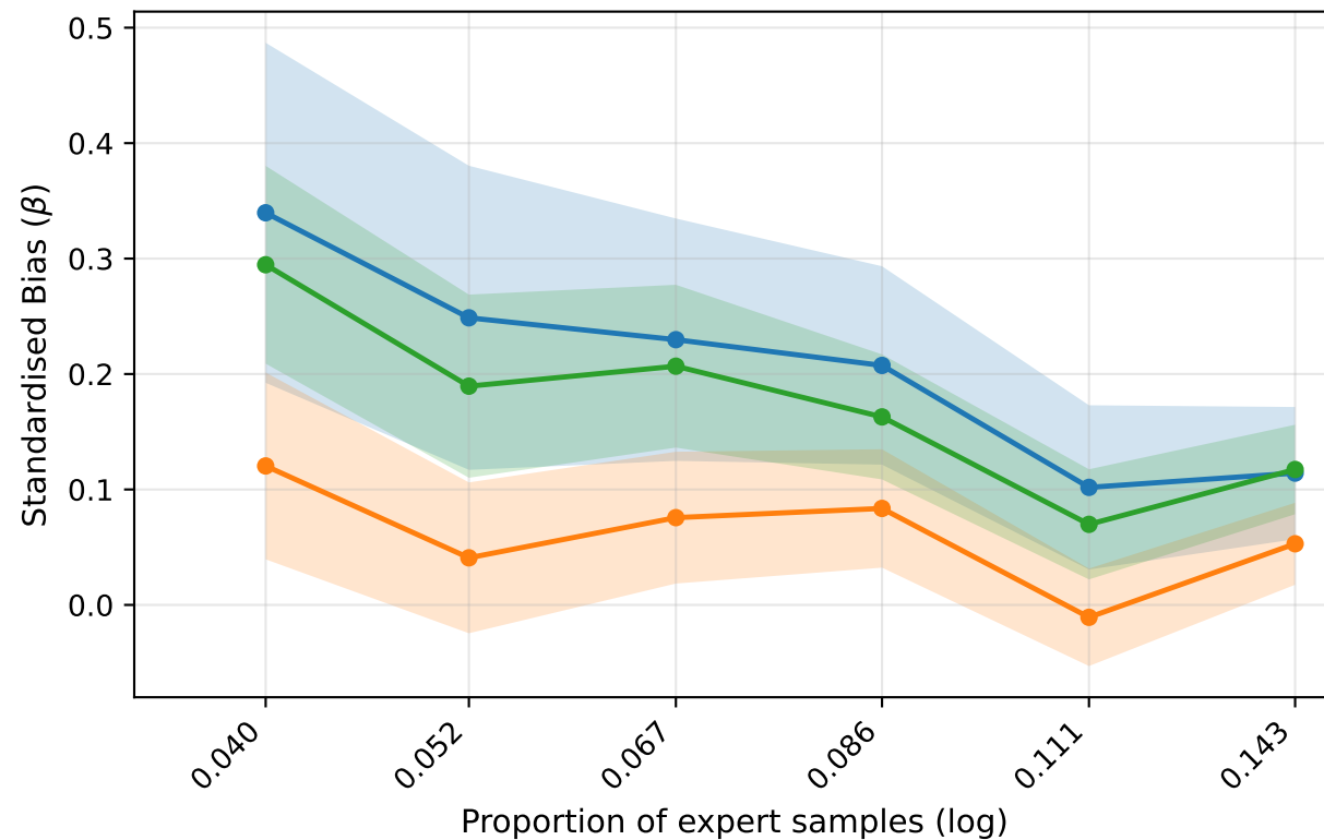
GPT-5.4
